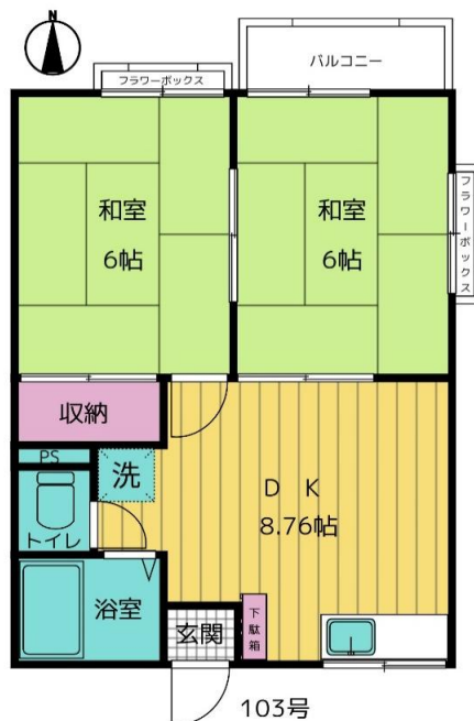
間取図
