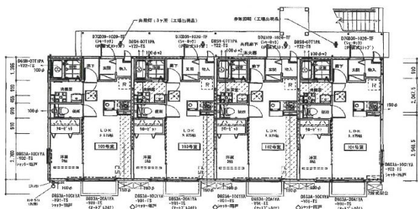
1階平面図
