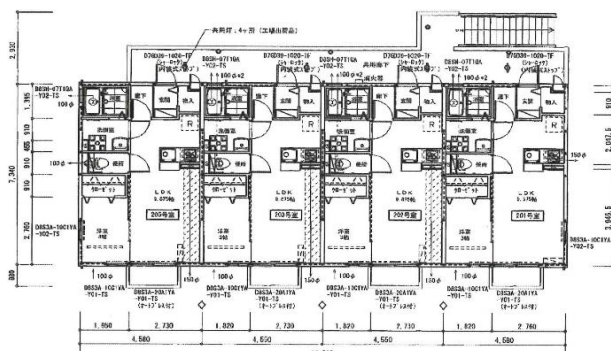
2階平面図
